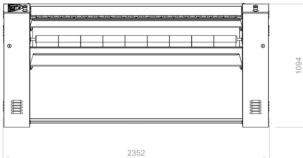
СПЕРЕДИ
