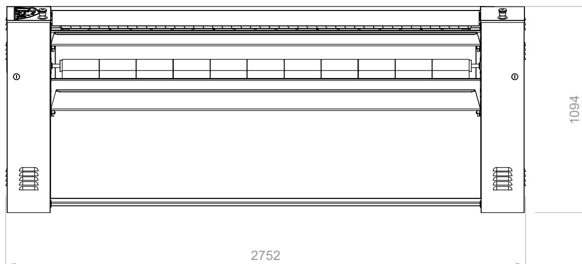
VUE FRONTALE
