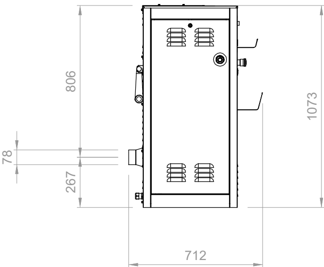
SEITENANSICHT
