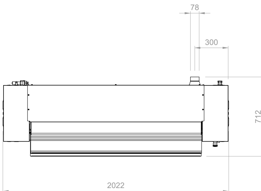
СВЕРХУ
