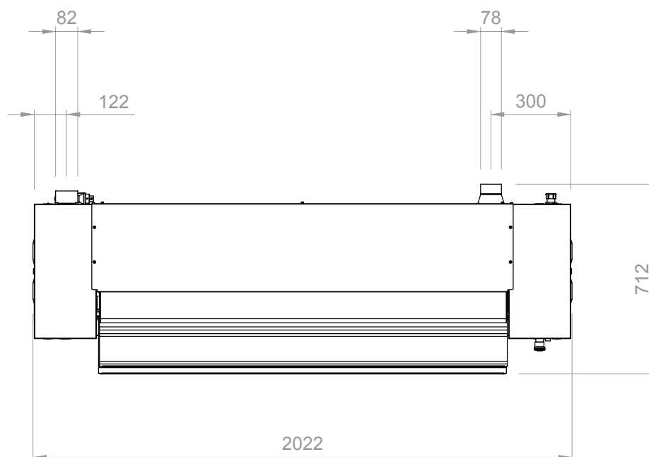
DRAUFSICHT
