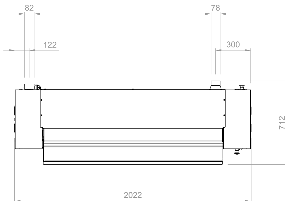
СВЕРХУ
