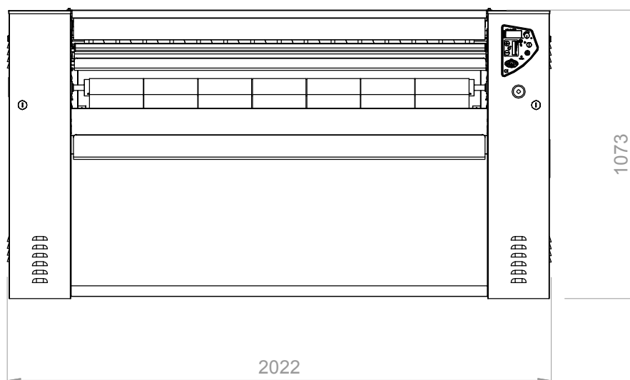
СПЕРЕДИ
