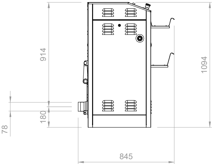
SEITENANSICHT
