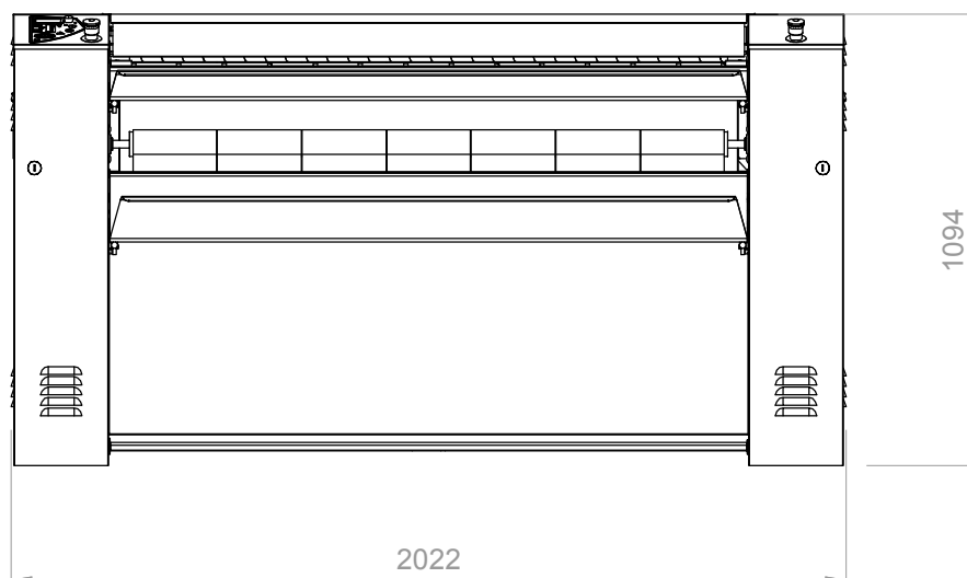
VUE FRONTALE
