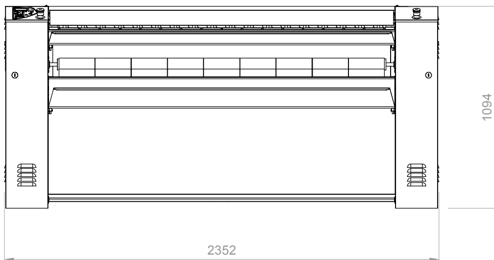
VISTA FRONTALE
