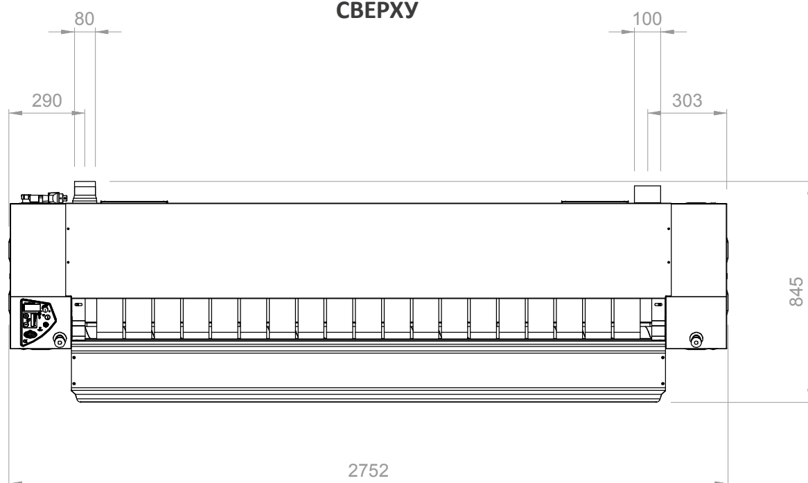
СВЕРХУ
