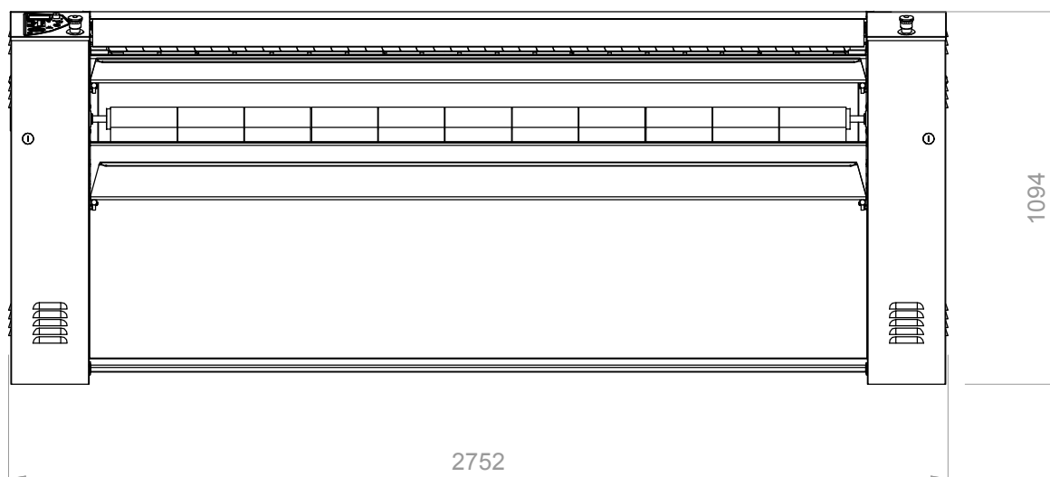
VORDERANSICHT
