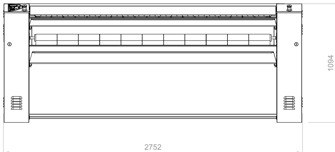
VISTA FRONTALE
