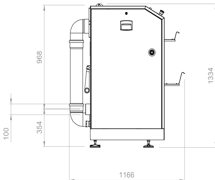
VISTA LATERALE
