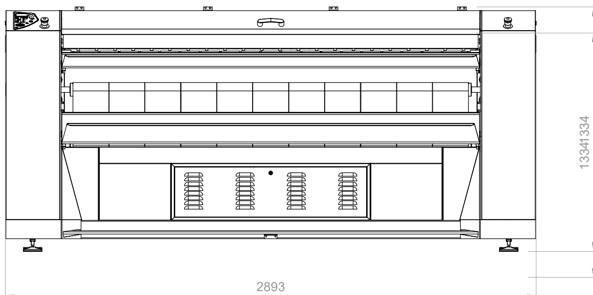
VISTA FRONTALE
