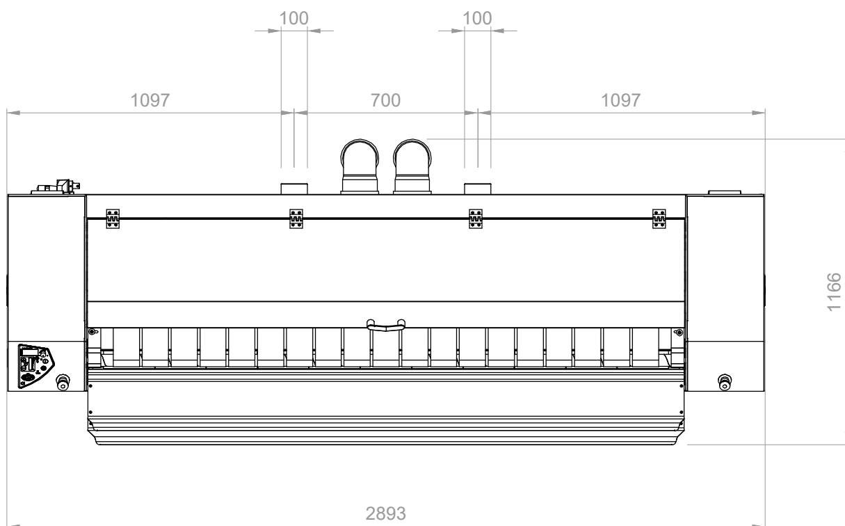
VISTA DALL'ALTO
