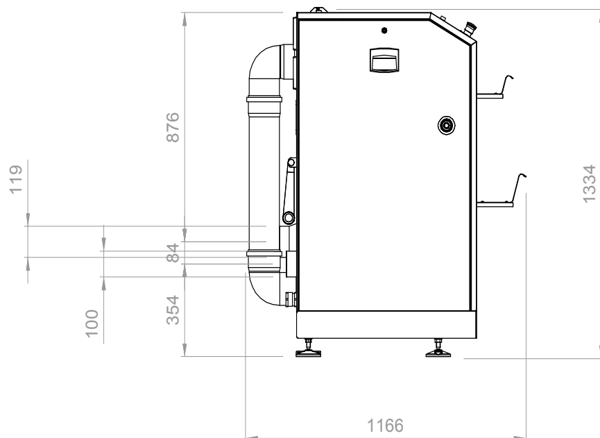
SEITENANSICHT
