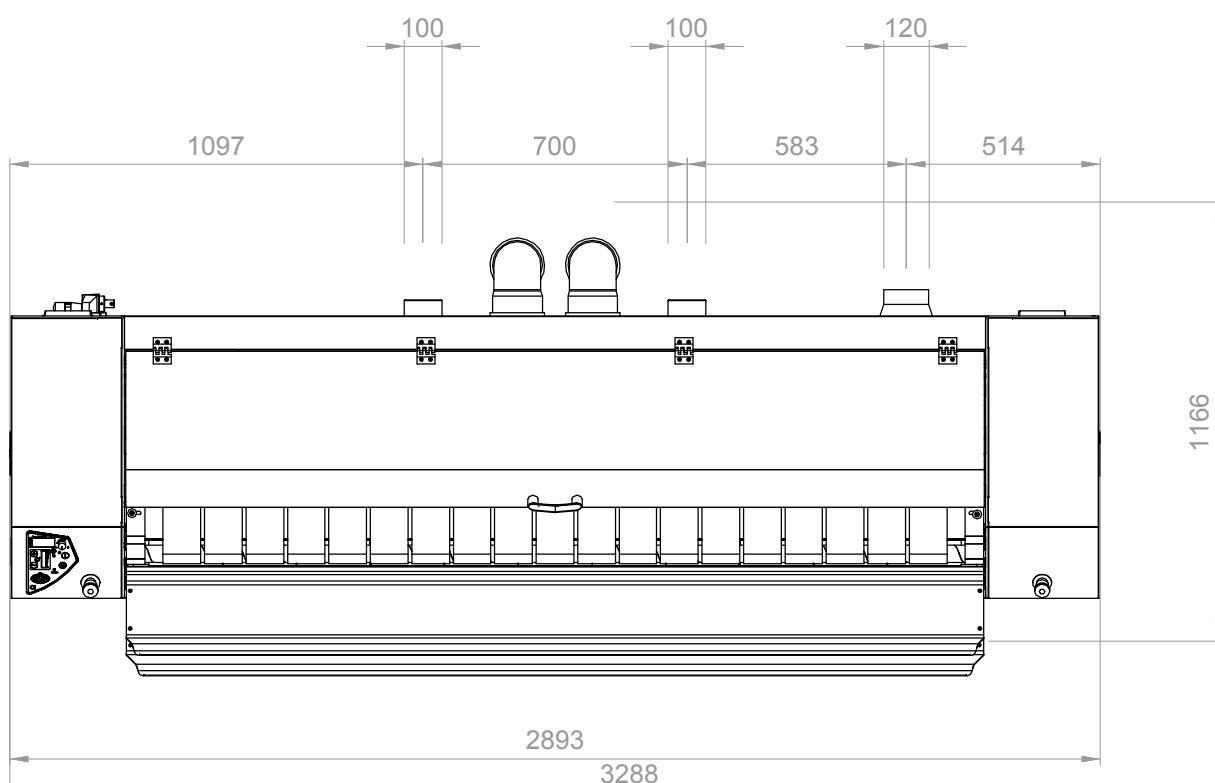
DRAUFSICHT
