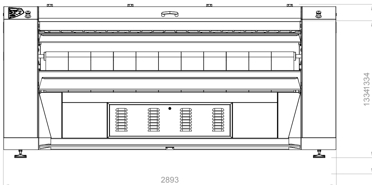
VORDERANSICHT
