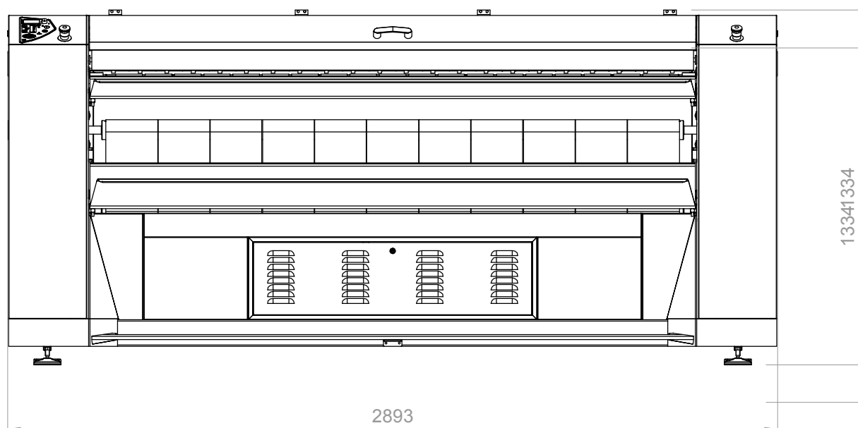
VUE FRONTALE
