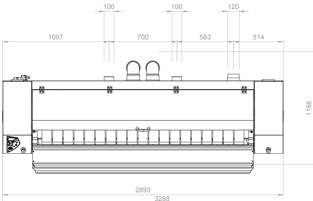
VISTA DALL'ALTO
