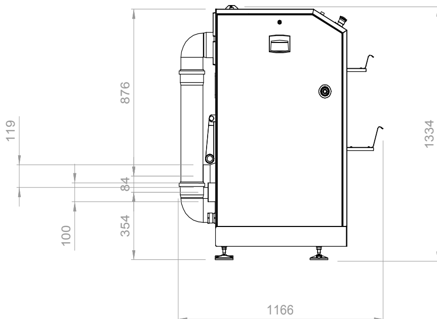
VISTA LATERALE
