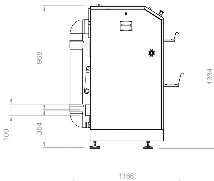
SEITENANSICHT
