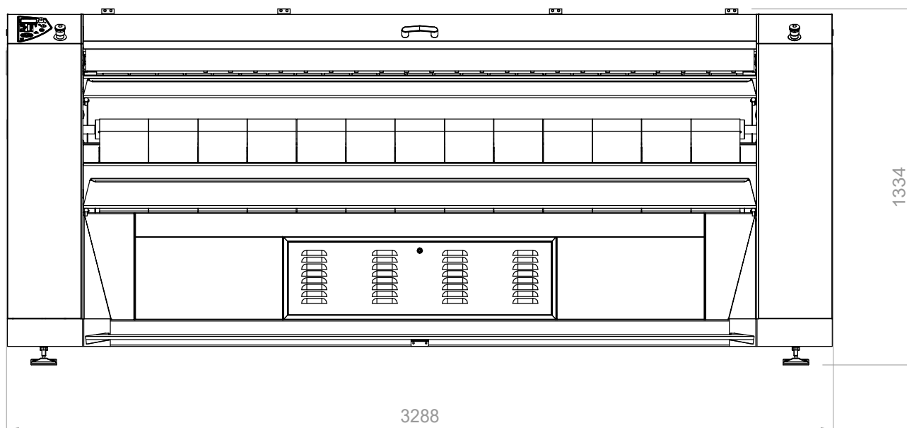
VORDERANSICHT
