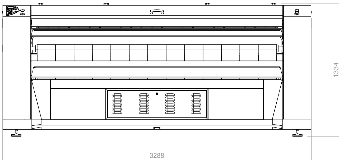
VUE FRONTALE
