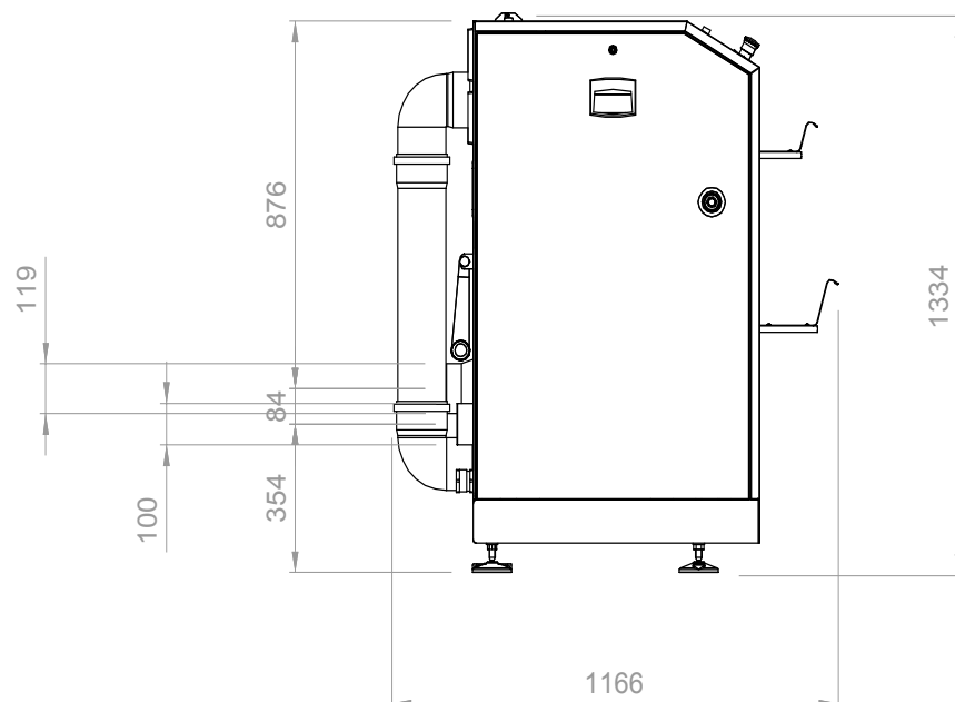
SEITENANSICHT
