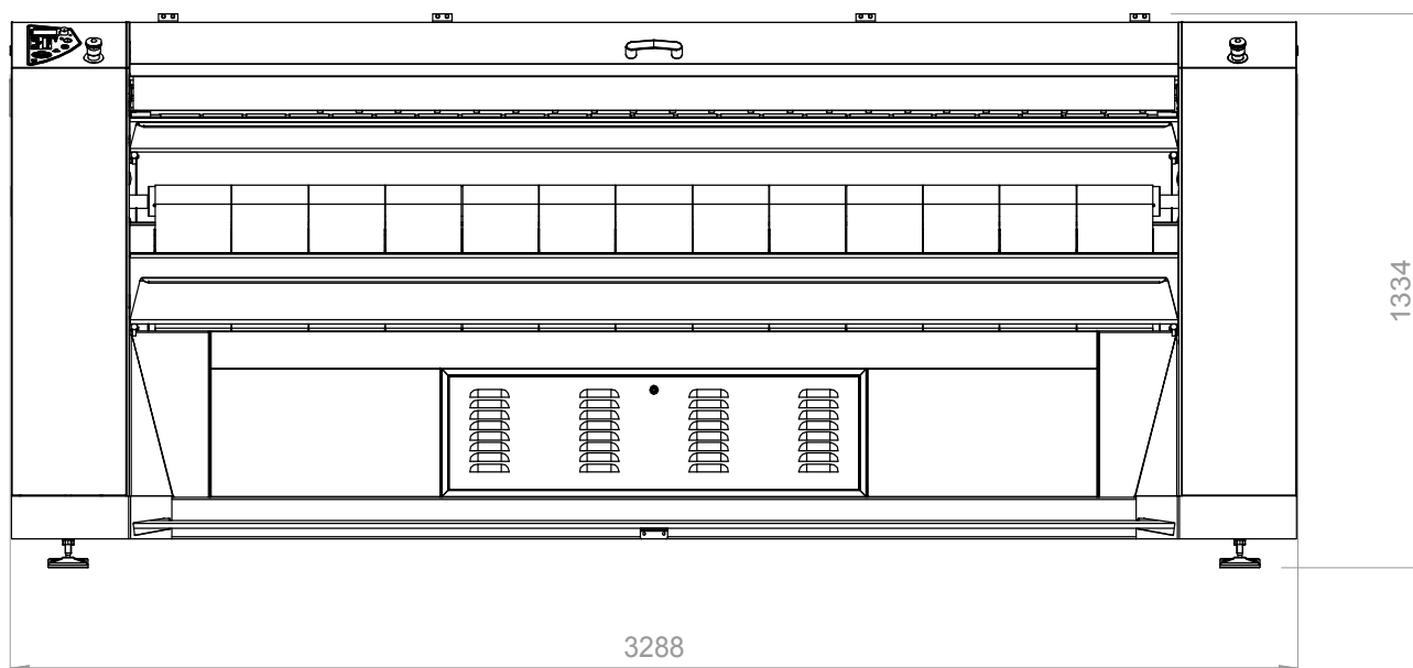
VORDERANSICHT
