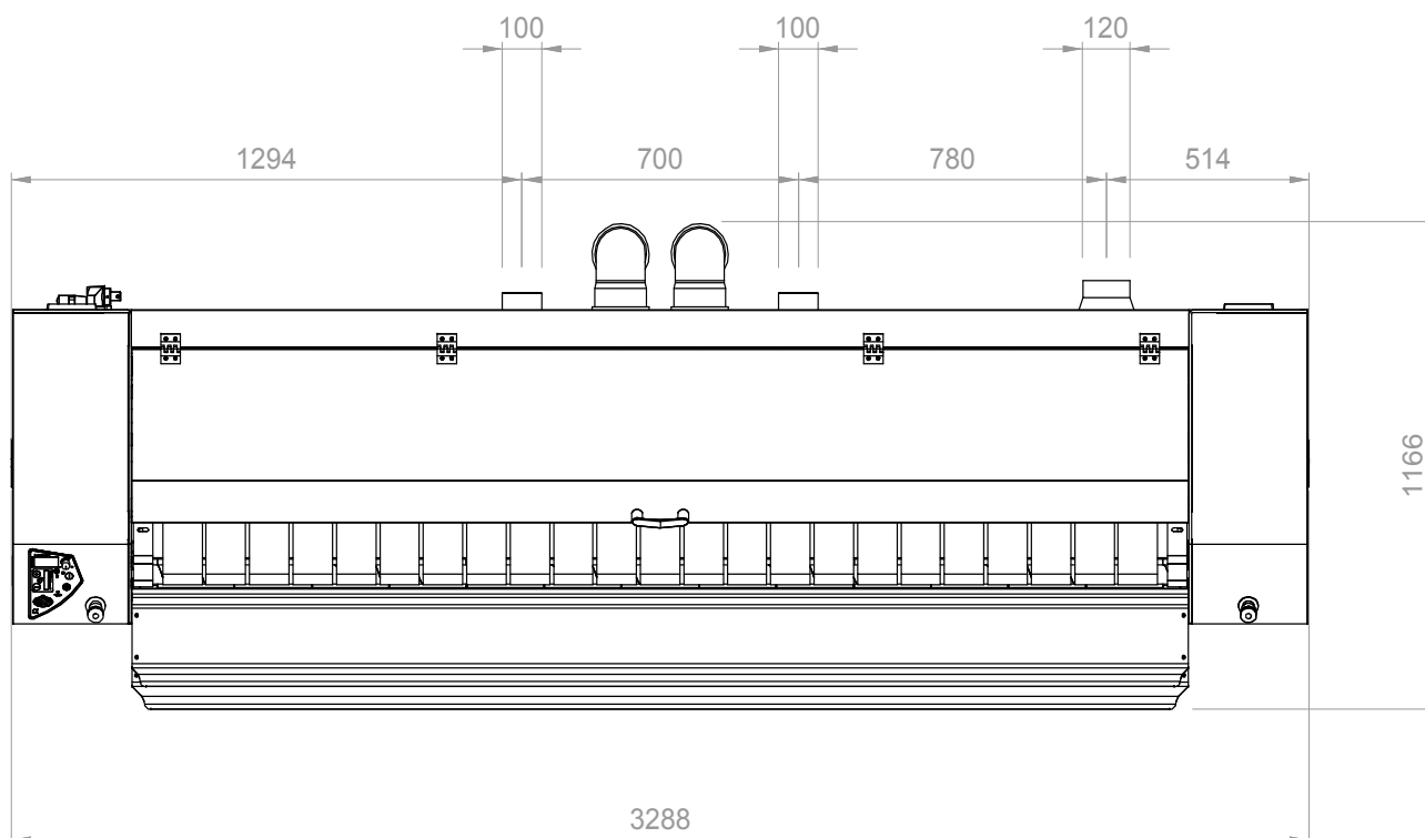
DRAUFSICHT
