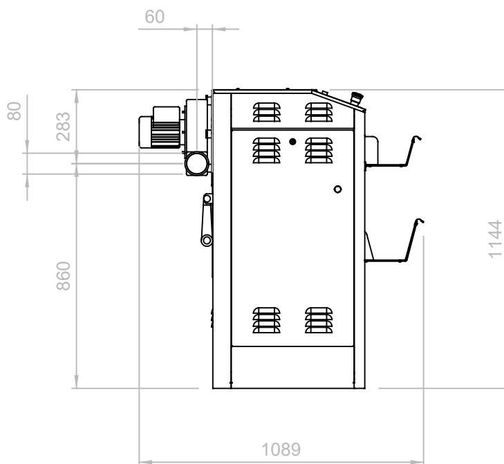
SEITENANSICHT
