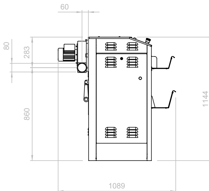
VISTA LATERALE
