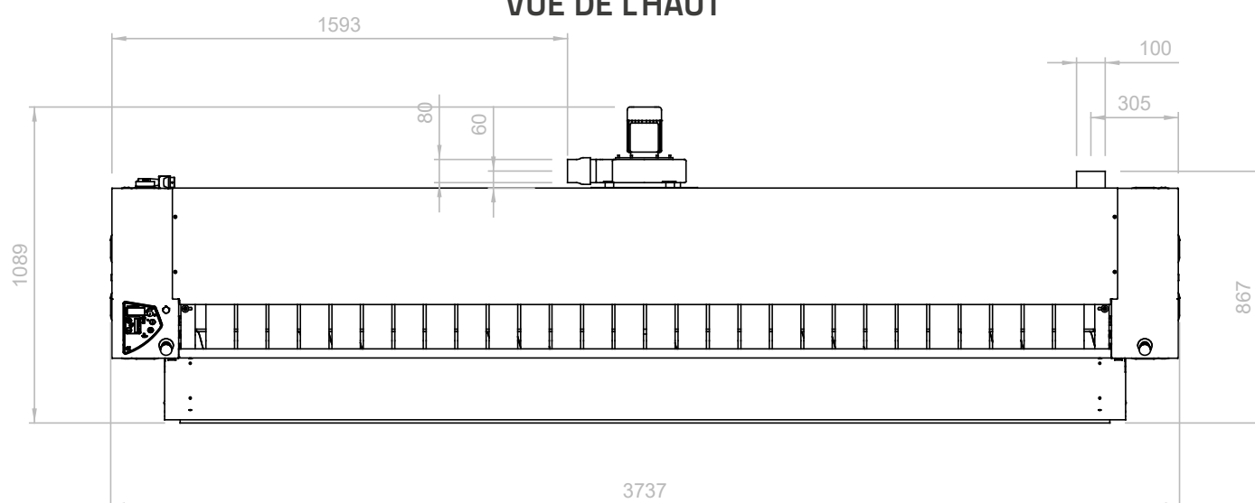
VUE DE L'HAUT
