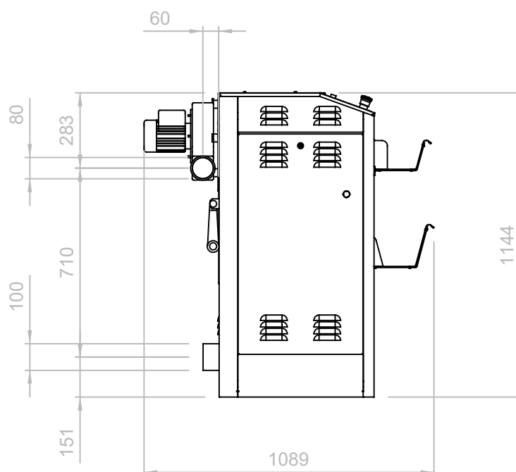
VUE DU CÔTÉ
