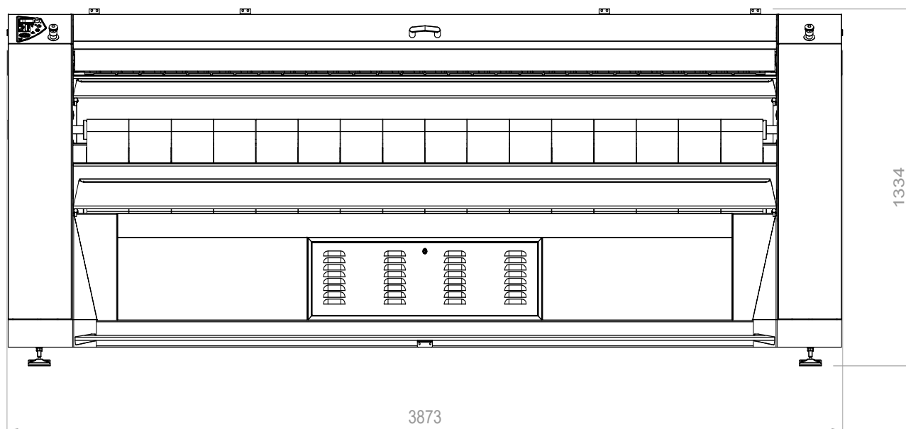
VORDERANSICHT
