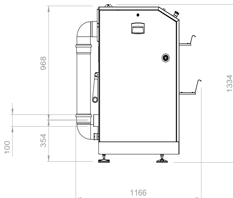
SEITENANSICHT
