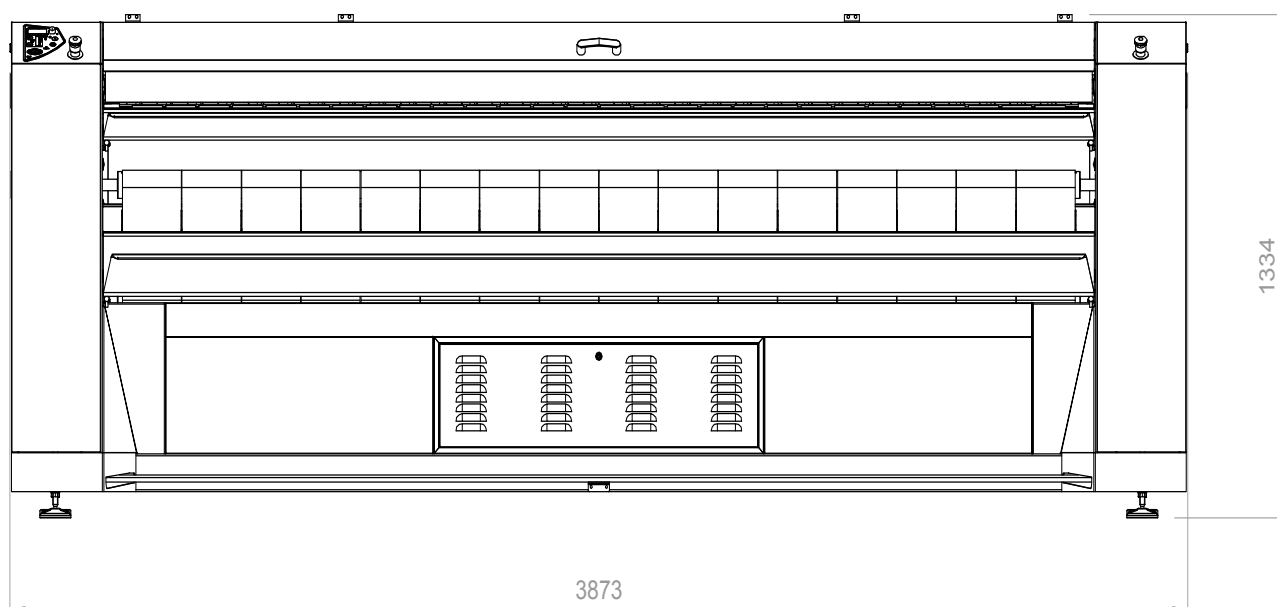
VORDERANSICHT
