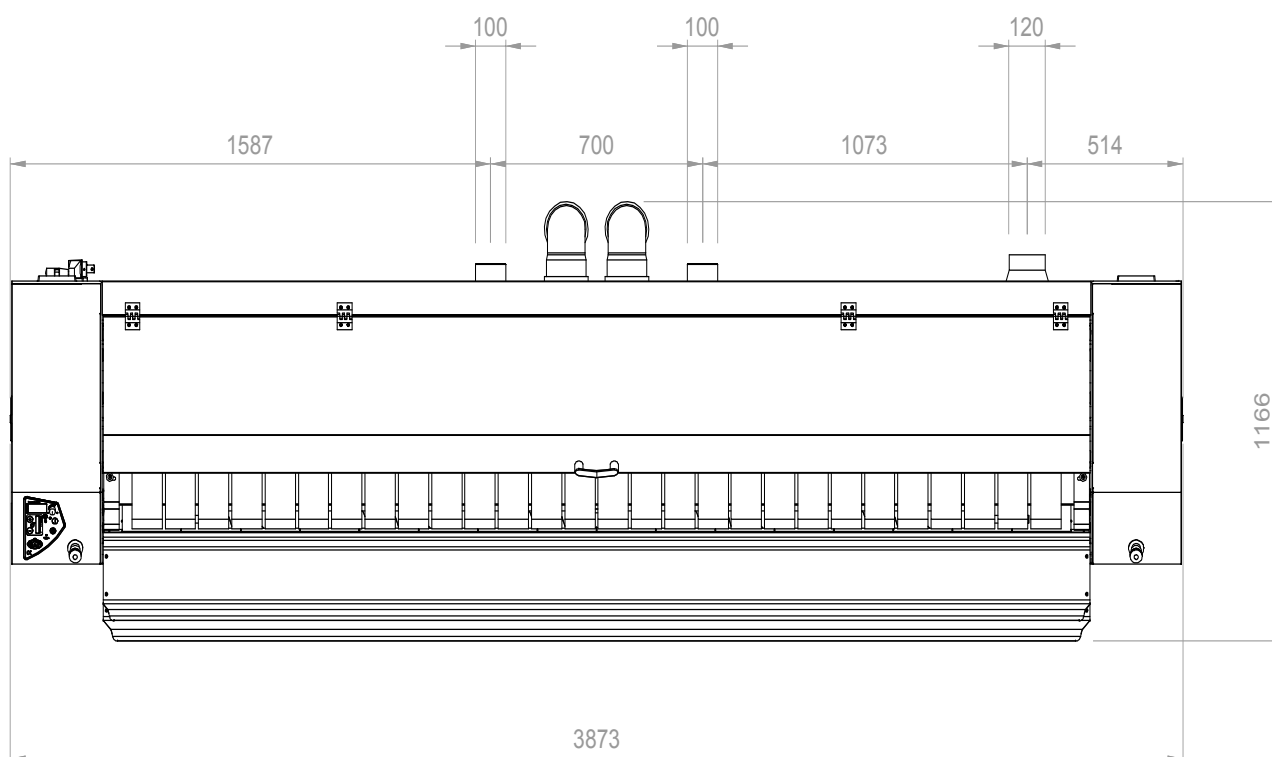
DRAUFSICHT
