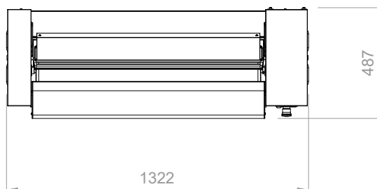
DRAUFSICHT
