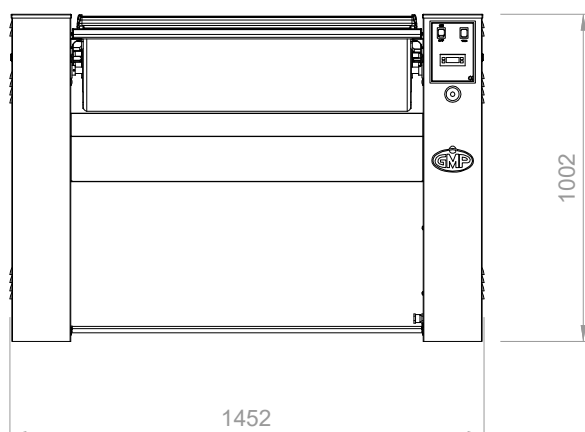
VISTA DALL'ALTO
