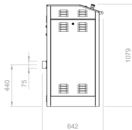
VUE DU CÔTÉ
