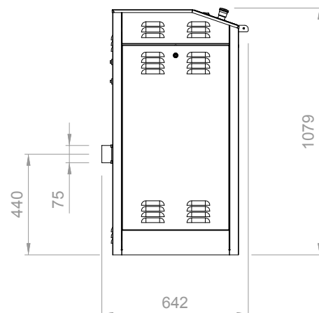
VUE DU CÔTÉ
