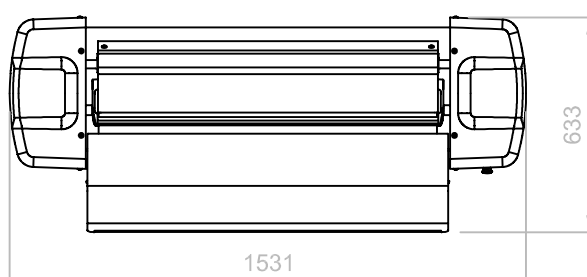
DRAUFSICHT
