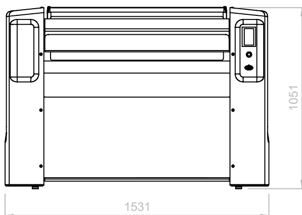
VORDERANSICHT
