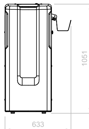
SEITENANSICHT
