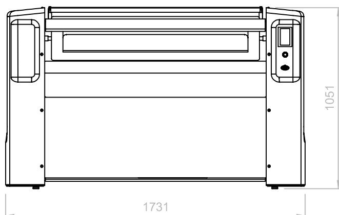
VUE FRONTALE
