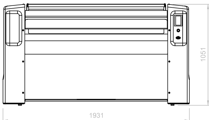
VORDERANSICHT
