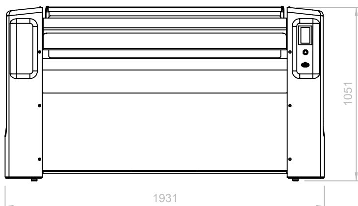
VISTA FRONTALE
