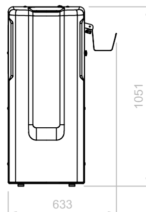
VISTA LATERALE
