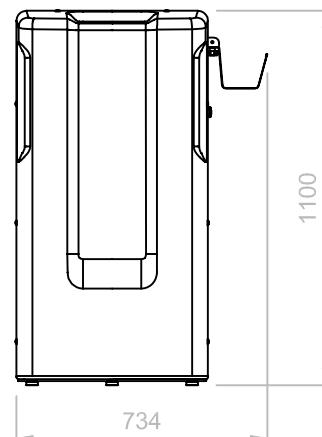
VISTA LATERALE
