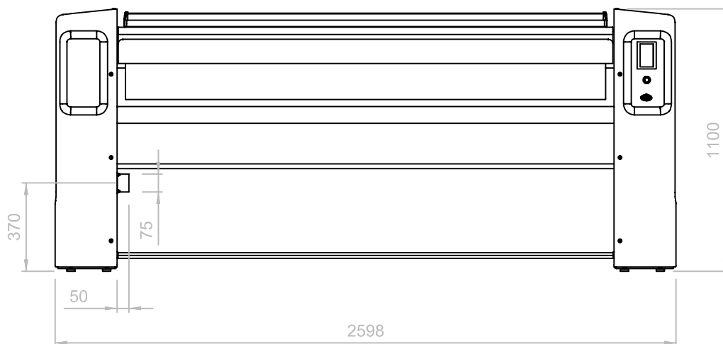
SEITENANSICHT
