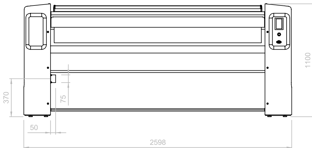
VISTA LATERALE
